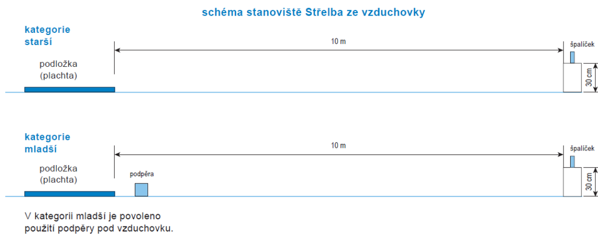
Obr. 1 Střelba – Schéma stanoviště střelba ze vzduchovky
